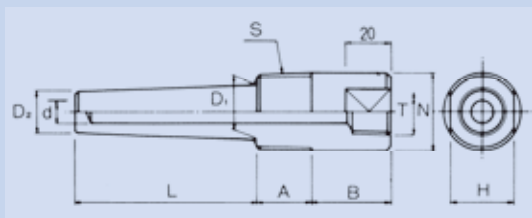
WL05 フランジ (ネジ込み) 形
