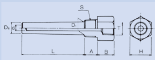
WL03 ネジ込み溶接形
