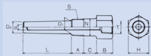
WL02 六角ネジ込み形
