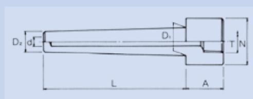
WL10 ヴァン・ストーン形
