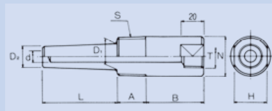
WL06 フランジ (溶接) 形
