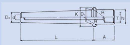
WL09 ポール・ジョイント形
