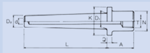
WL10 ヴァン・ストーン形
